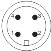
RTD 与圆形连接器连线图
