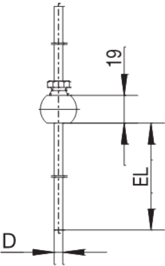
卡箍符合 DIN 32676 标准
