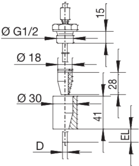
带紧固螺母的卡箍 DIN 11851（牛奶管接头）
