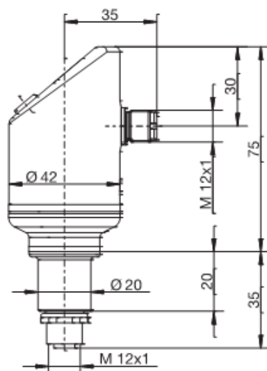
型号：902940/50 带 M 12x1 连接 RTD 温度探头
