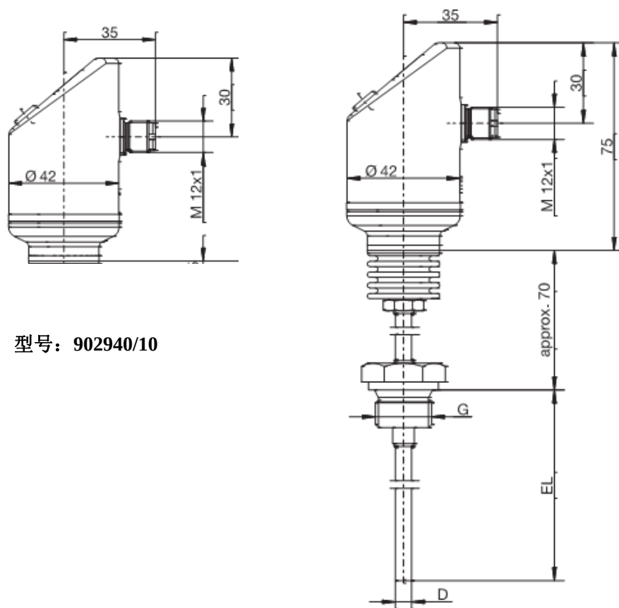
型号：902940/30 带延长管
